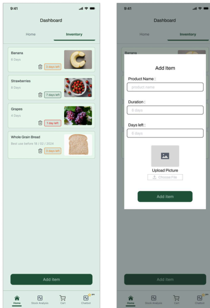
Wireframe 2. Wireframe fitur inventory
