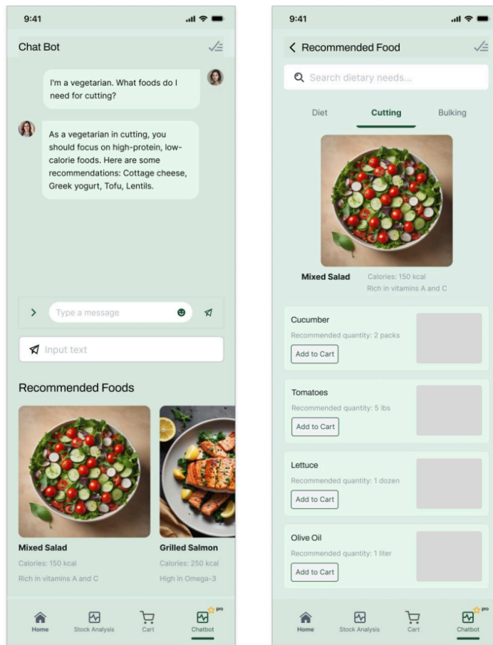
Wireframe 3. Wireframe fitur chatbot
