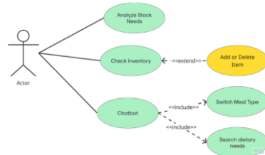
Gambar 3. Use Case Keseluruhan Aplikasi
