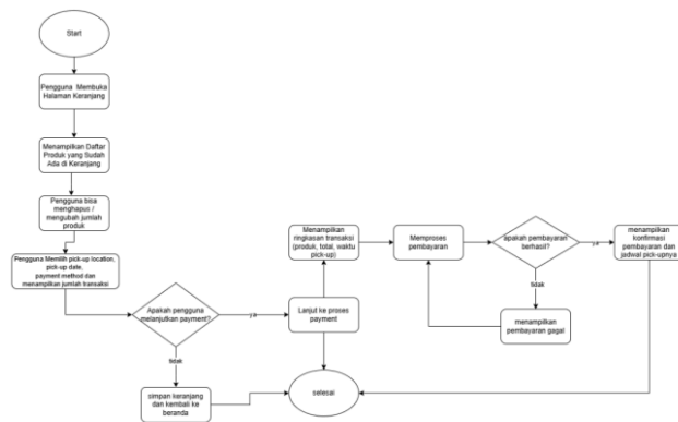
Flowchart 2. Flowchart fitur keranjang dan transaksi
