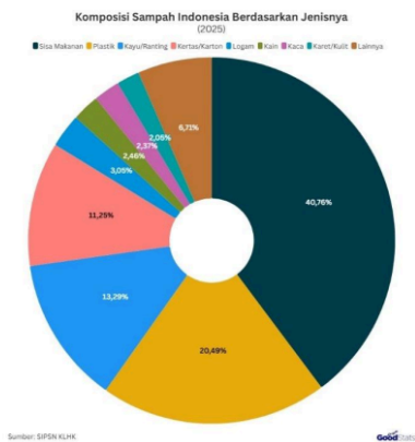
Gambar 1. Komposisi sampah berdasarkan jenis sampah
